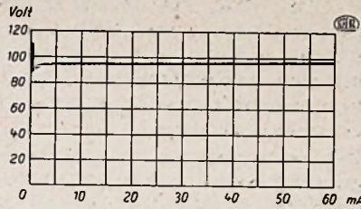
Fig. 6. — Stroom-spanningscurve van een glimlichtbaan.
