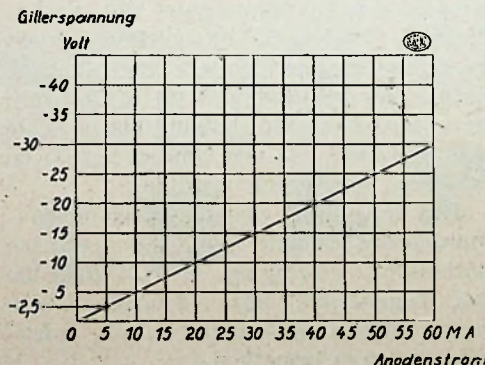
Fig. 3. — Verband tusschen anodestroom en negatieve roosterspanning, wanneer het gewone plaatstroomapparaat die automatisch levert.
