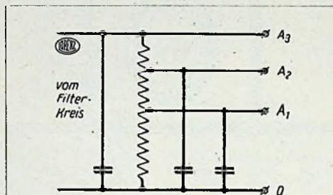
Fig. 2. — Spanningsverdeling door een potentiometer van weerstanddraad.
