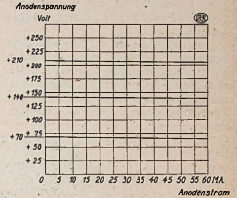
Fig. 8. — Curven, die het verband tusschen spanning en stroomafname van een plaatstroomapparaat met glimlicht spanningsdeeler aangeven.
