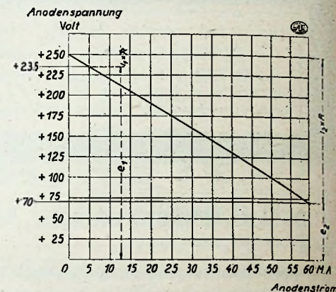
Fig. 4. — Verband tusschen spanning van het gewone plaatstroomapparaat en grootte der stroomafname. De spanning daalt snel.
