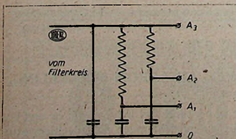
Fig. 1. — Tot dusver gebruikelijke spanningsregeling met serie-weerstanden.
