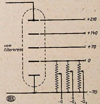
Fig. 9. — Hoe de roosterspanning met gewone potentiometers wordt onderverdeeld. De spanningen zijn onafhankelijk van den plaatstroom.
